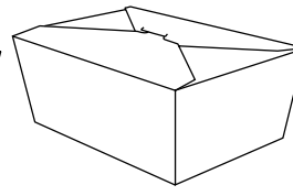
TTPLA-4 84oz 7.76" x 5.51" x 3.54" 160/cs 3.71/cu.ft
